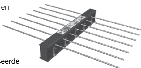
HALFEN HIT-HP/SP MV Koudebrugonderbreking
