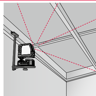
... Decken abhängen
